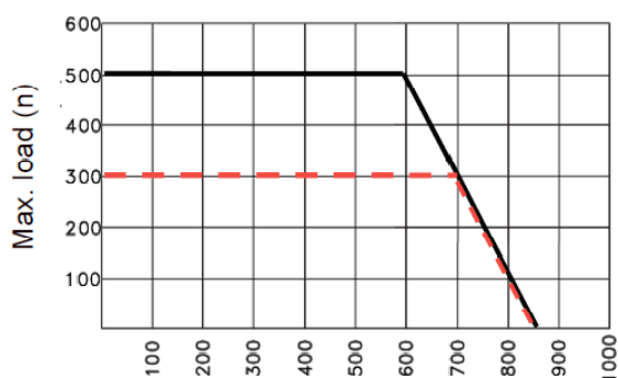
Максимальная нагрузка цепи (Н) в зависимости от выхода цепи (мм)
